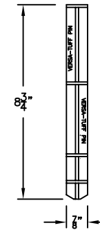
VERSA-LOK BRUTE PIN SCALE: NONE
